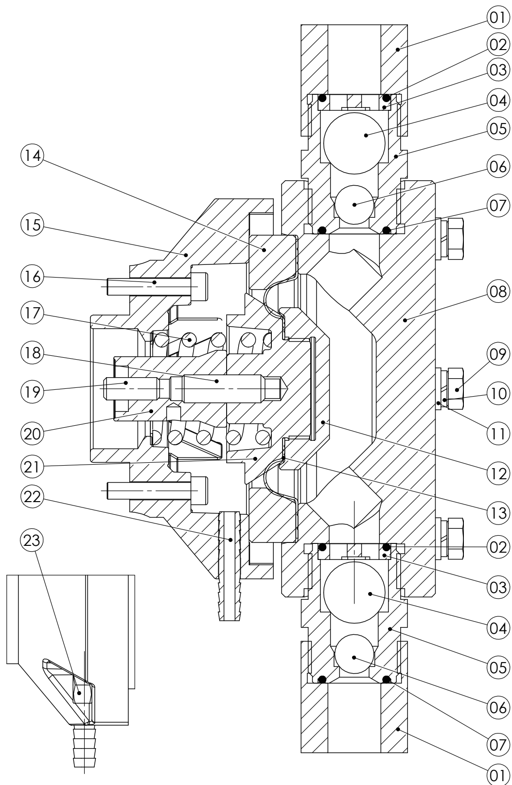
图 10 NPBG0090-NPBG0500 不锈钢液力端
