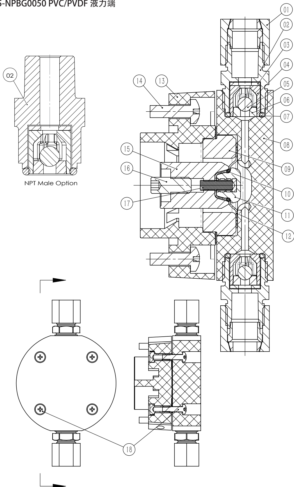
图 7 NPBG0025-NPBG0050 PVC/PVDF 液力端
