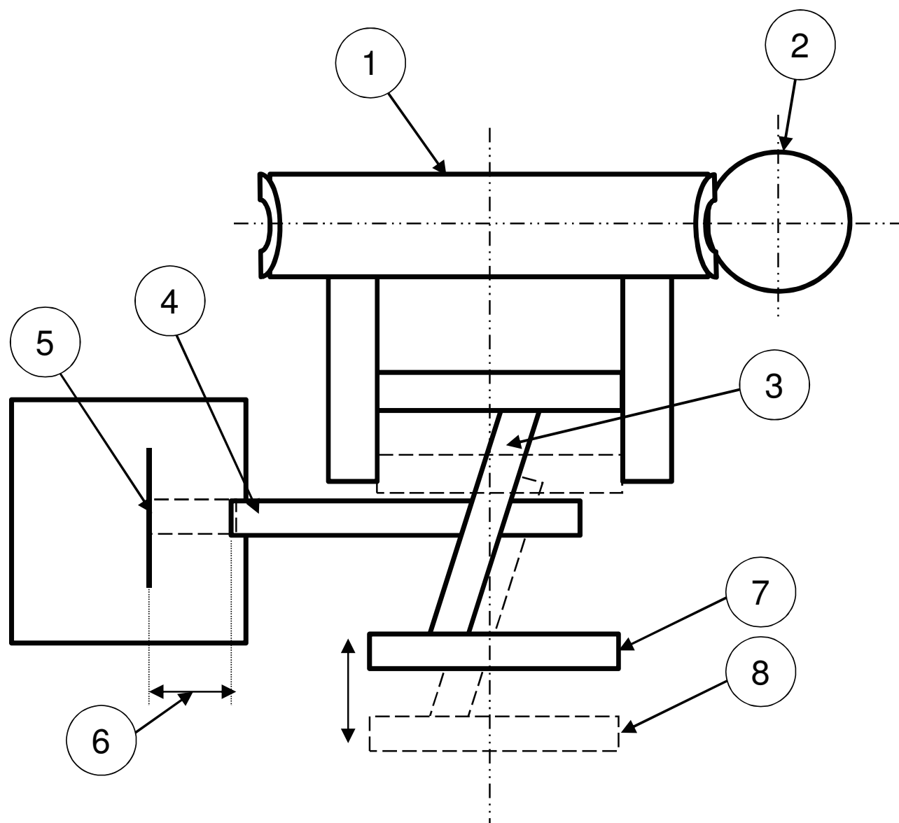
图2：冲程调节原理
