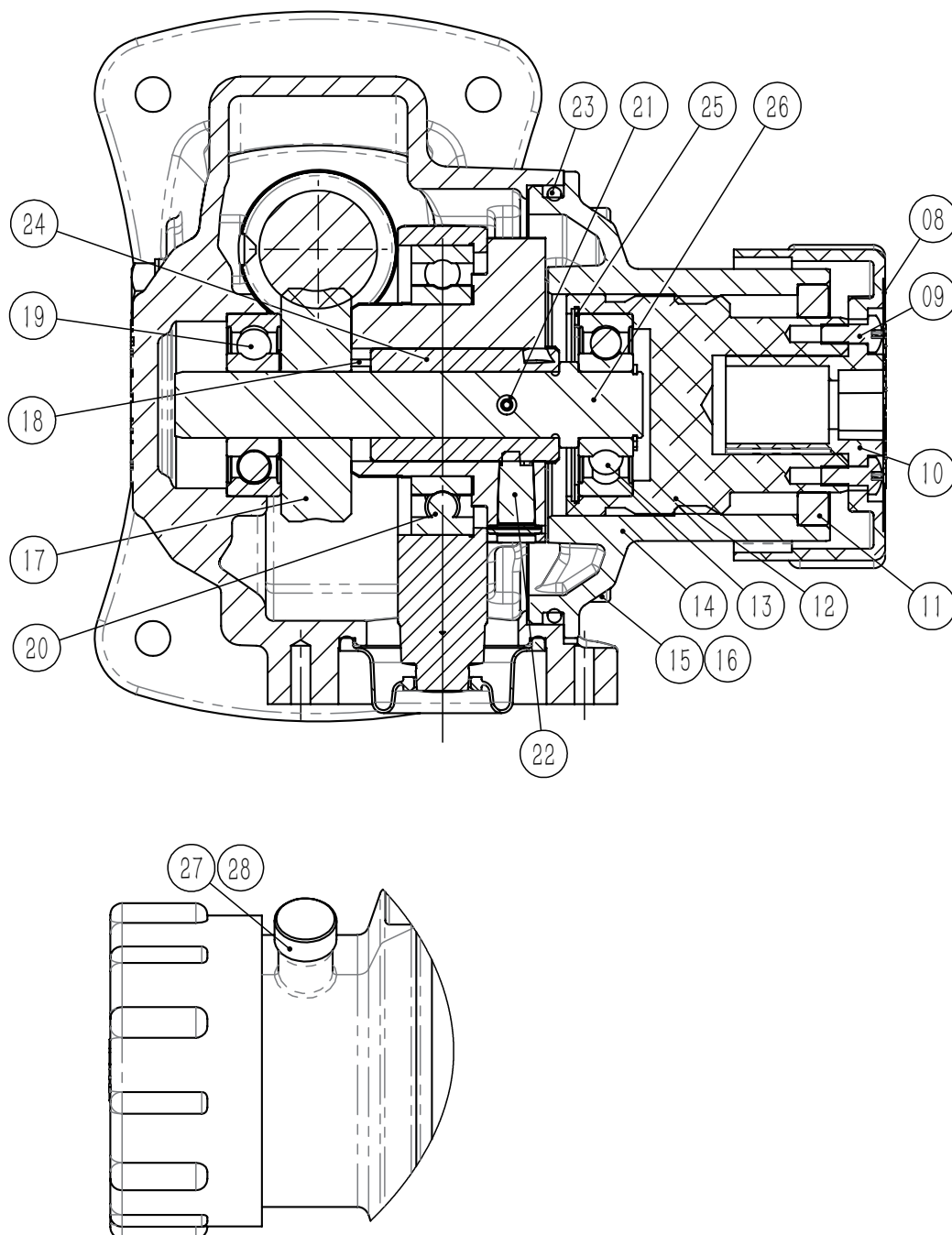
图 6 NPBG 驱动端 (端面图)
