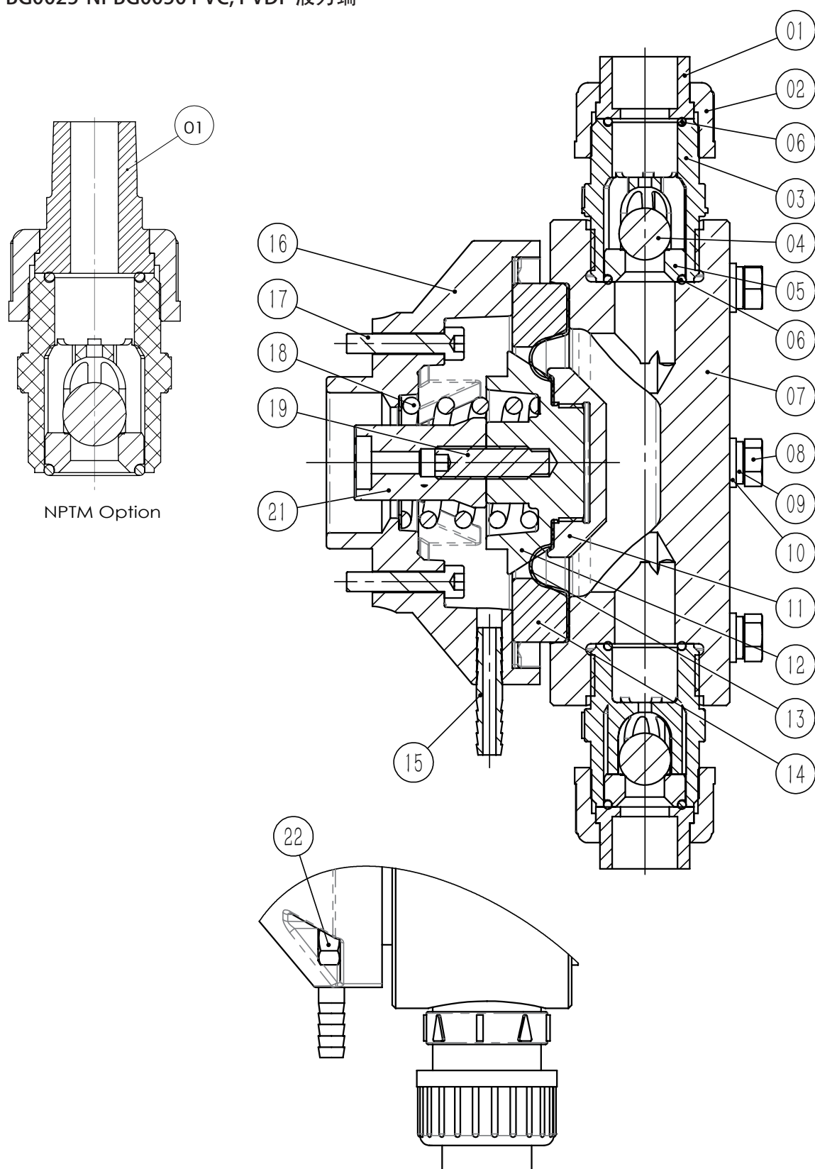
图 8 NPBG0025-NPBG0050 PVC, PVDF 液力端
